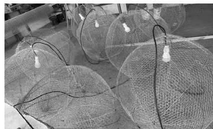
Estrutura das bolas em arame.
